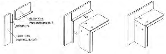
Рис. 18 Установка наличников под прямым углом.
